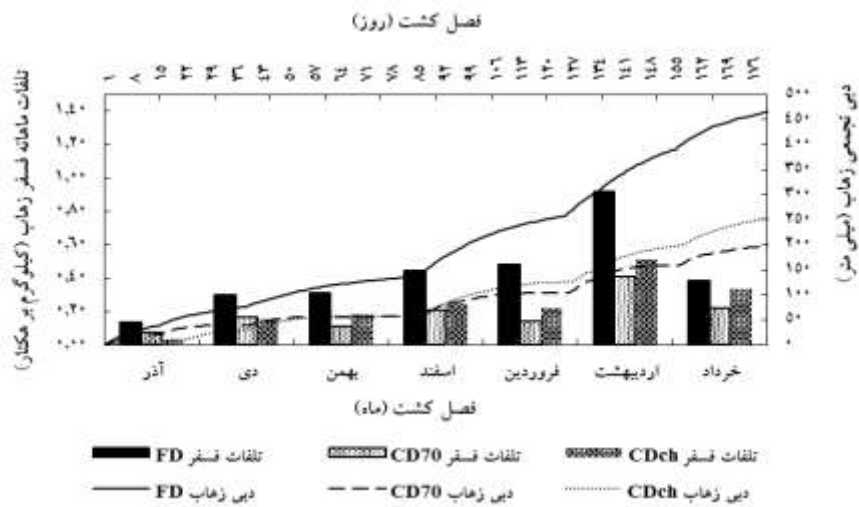
شکل ۶. تلفات ماهانه فسفر و حجم زهاب تجمعی محصول جو
