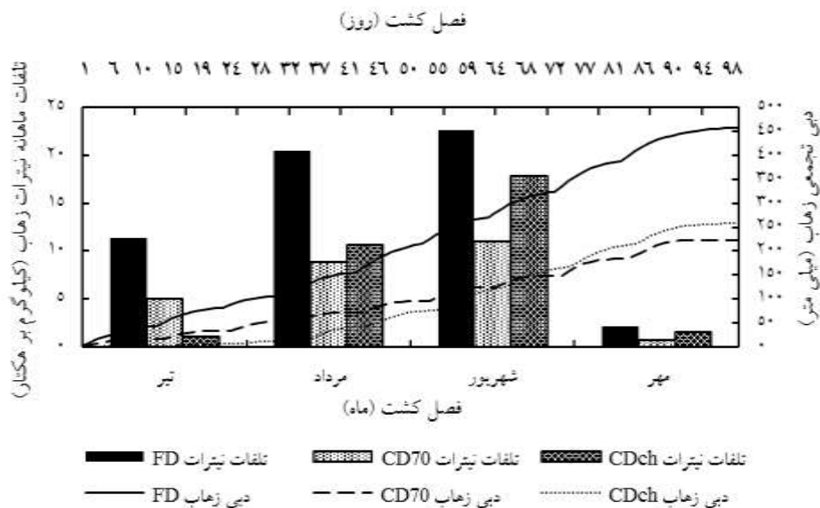
شکل ۵. تلفات ماهانه نیترات و حجم زهاب تجمعی محصول ذرت
