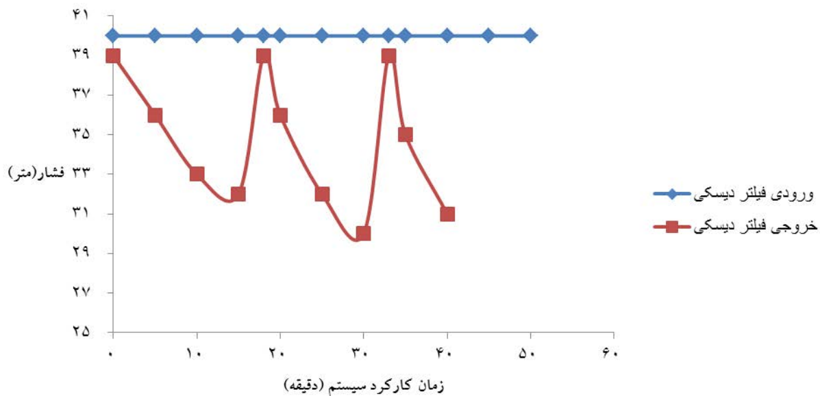
شکل ۵. زمان گرفتگی فیلترهای دیسکی، بدون حضور تانک شن در کیفیت آب آبیاری با محدودیت شدید
