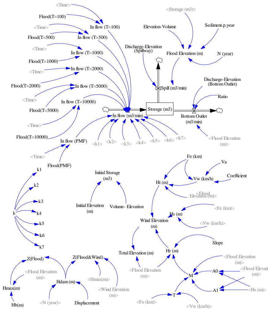
شکل ۴. نمایی از مدل ساخته شده برای شبیه سازی سطح آب مخزن سد حاجیلرچای و محاسبه تابع عملکرد سیستم
