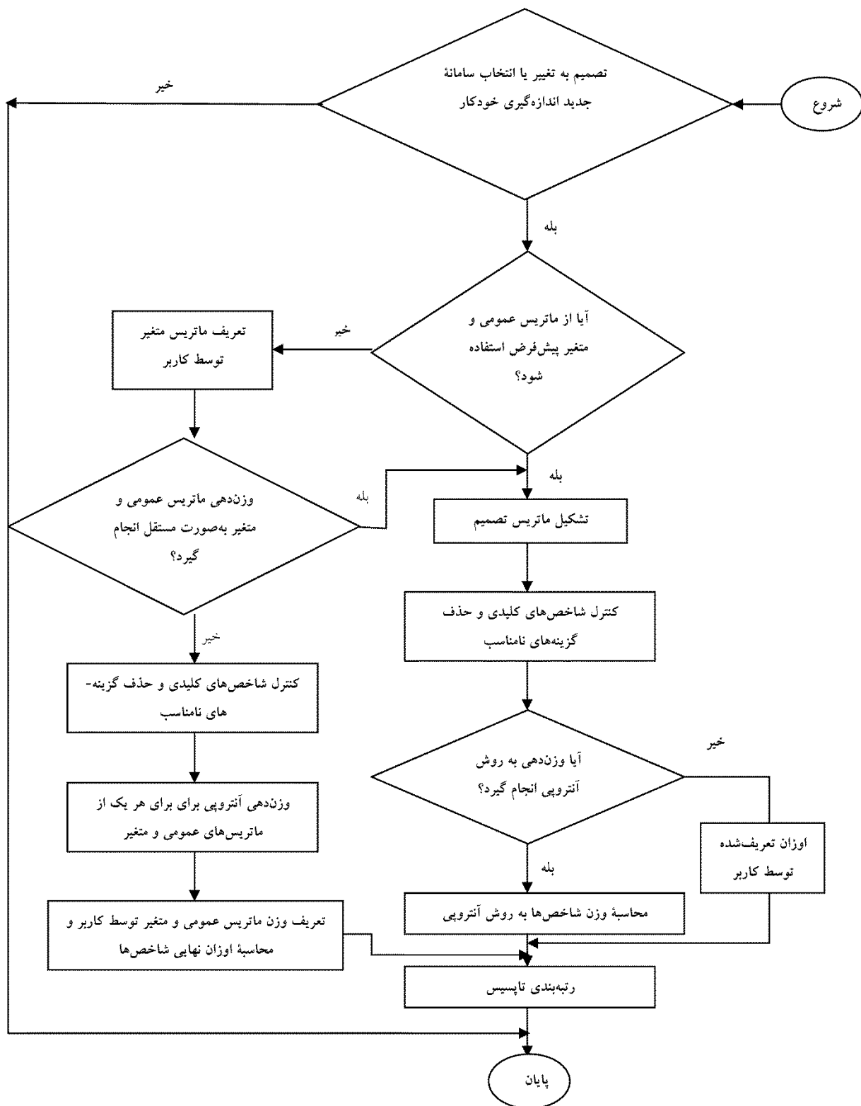
شکل ۱. نمودار گردش برنامه روش تاپسیس برای انتخاب گزینه های مختلف سامانه های خودکار اندازه گیری
